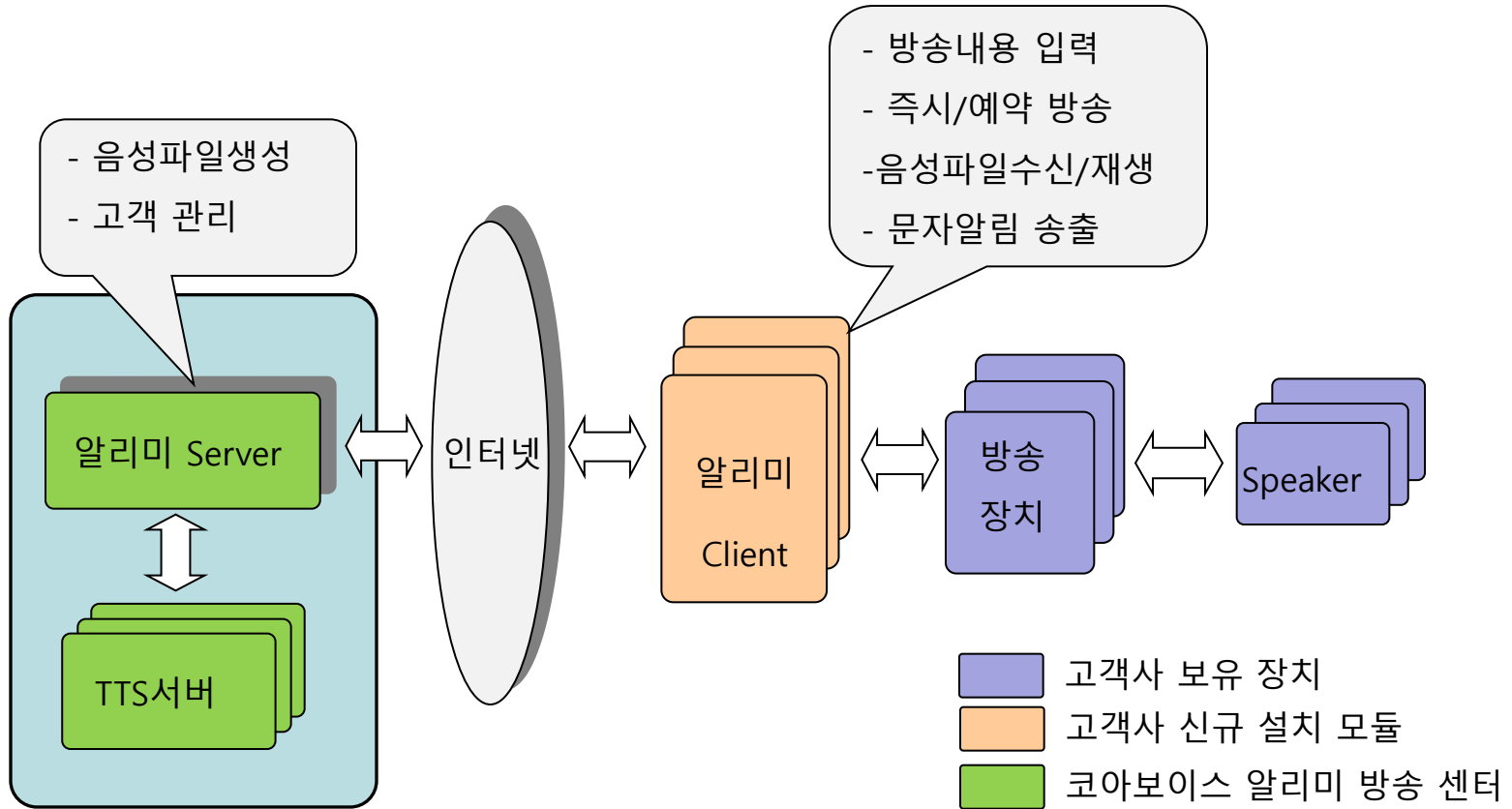
[그림] 인터넷기반 알리미 방송 시스템 구성도
