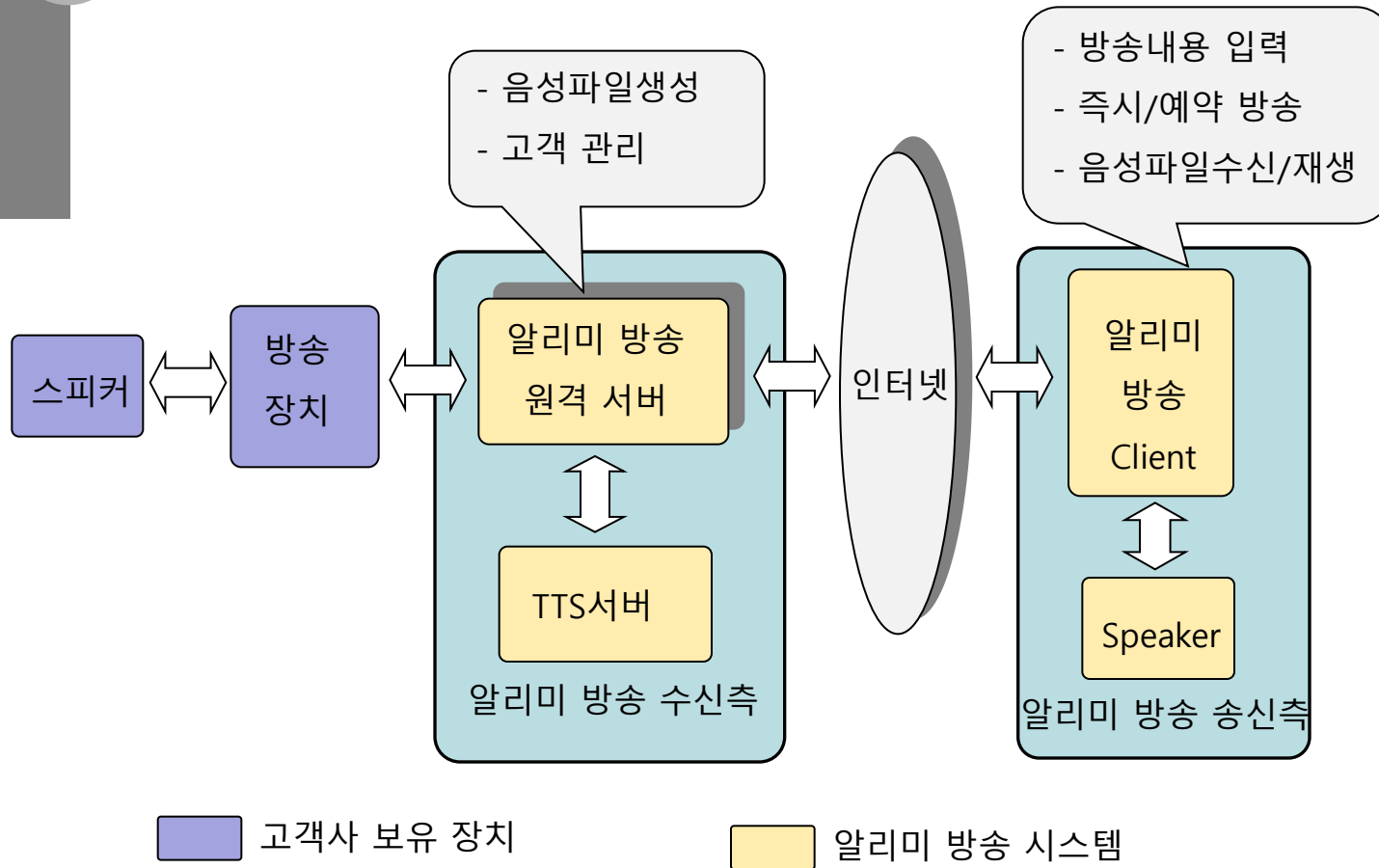
[그림] 알리미 원격 방송 시스템 구성도
